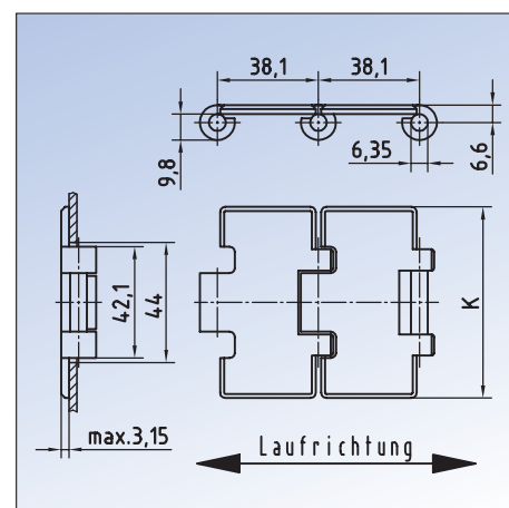
Geradgängig: Einfach-Scharnier, 38,1 mm Teilung
