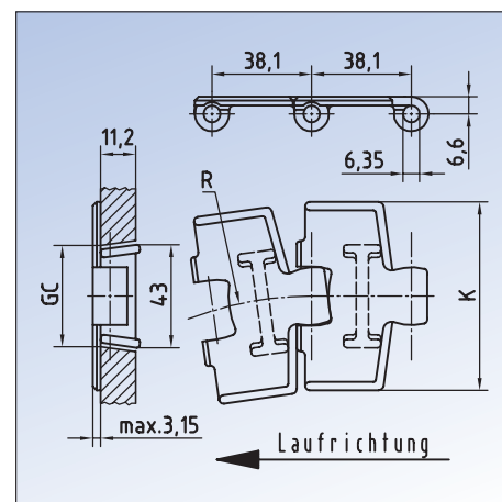
Kurvengängig: 38,1 mm Teilung, Schwalbenschwanz-Führung
