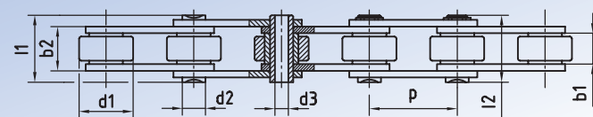
Hohlbolzenkette mit Laufrollen
